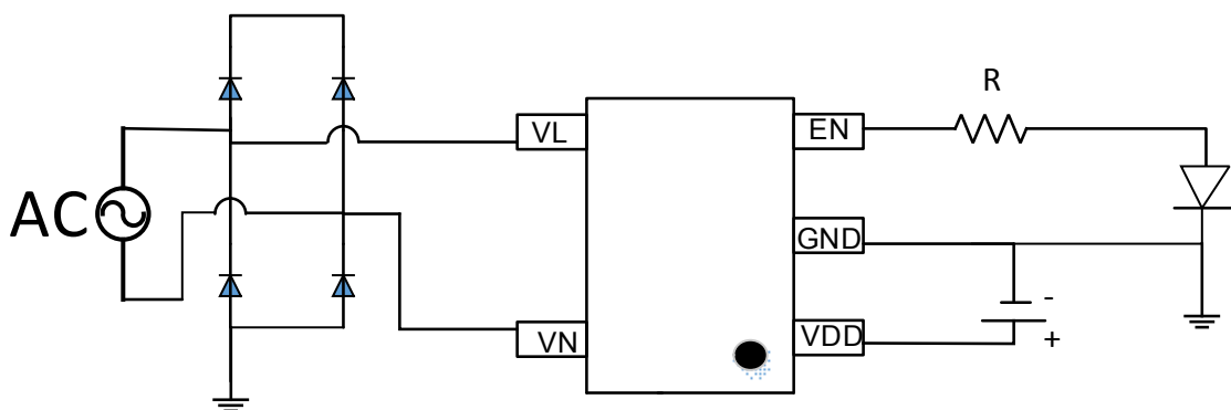
图一 QW2881 典型应用电路
